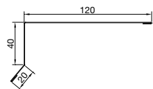
Vindskiva TP Längd: 2 000 mm Täckande: 1 900 mm
